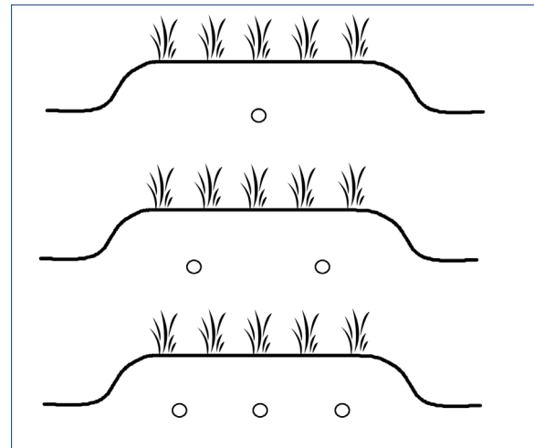
Figura 1. Esquema de varias configuraciones de cintas de riego por goteo subterráneas usadas para la producción de cultivos.
